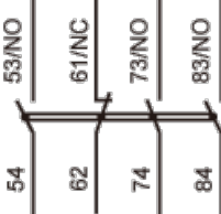
3NO+1NC(LANN31)
