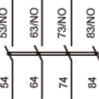
4NO(LANN40)
