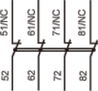
4NC(LANN04)
