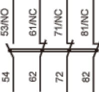
1NO+3NC(LANN13)
