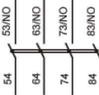
4NO(LANN40)
