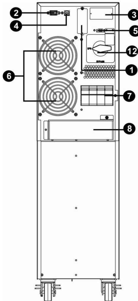
图 2: 3/1 15K/20K 背面面板
