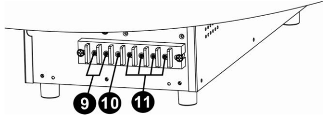
图 4: 3/1 10K(L) 输入输出端子
