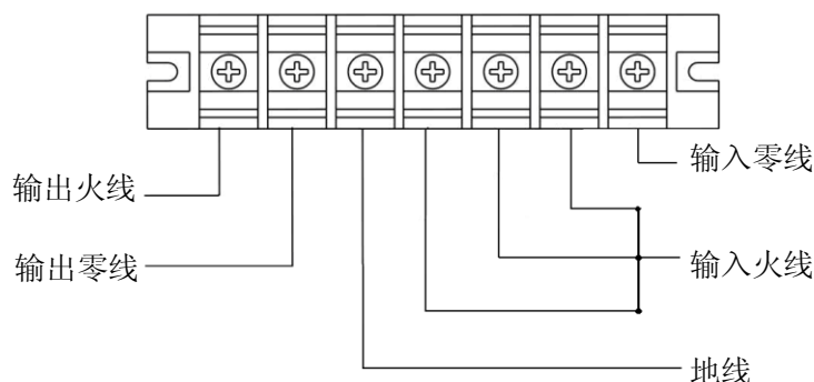
端子台示意图（单相输入）
