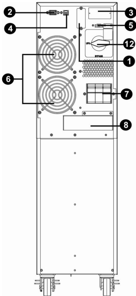
图 1: 3/1 10K 背面面板
