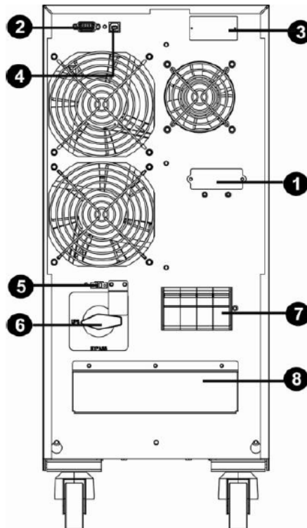
图 2: 3/1 15KL 背面面板
