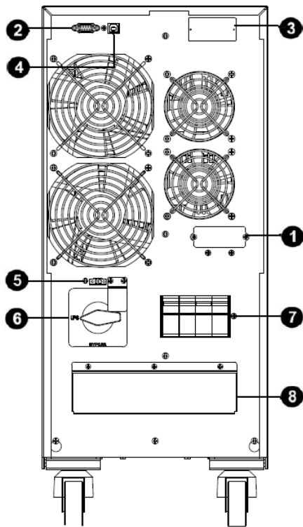
图 3: 3/1 20KL 背面面板
