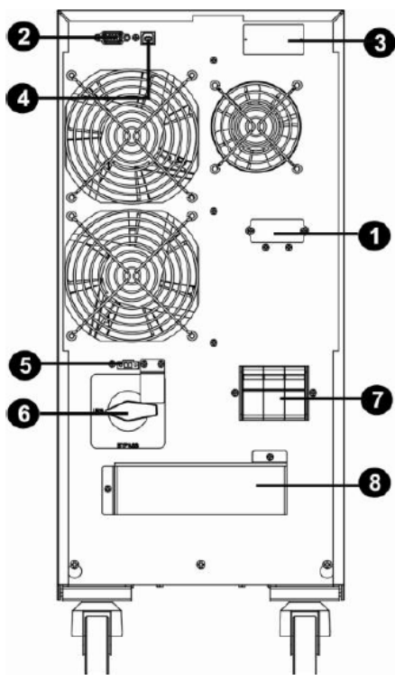
图 1: 3/1 10KL 背面面板
