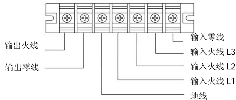
端子台示意图
