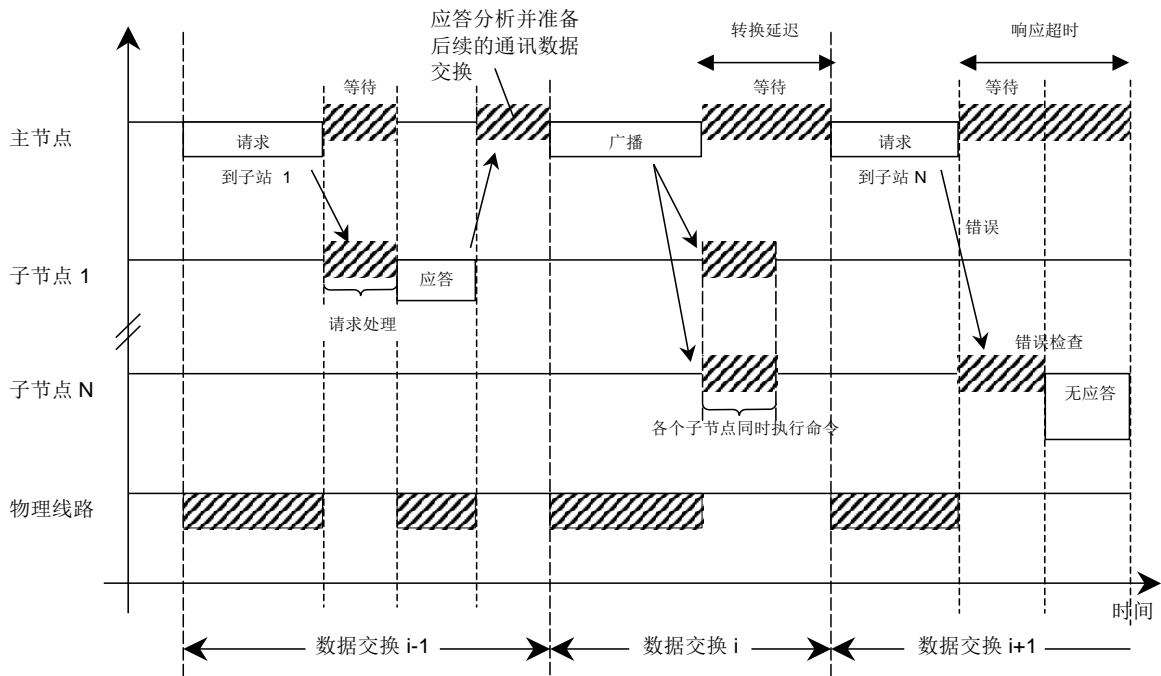
图 9: 各种情形的主/从通信时序图
