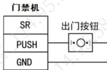
图4-1 连接示意图
