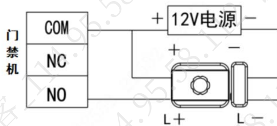
图1-23 接线示意图
