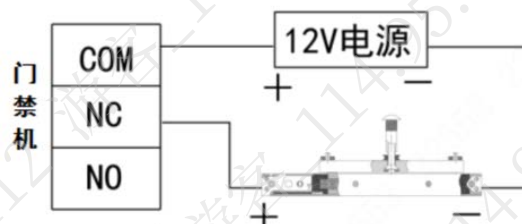
图1-9 接线示意图
