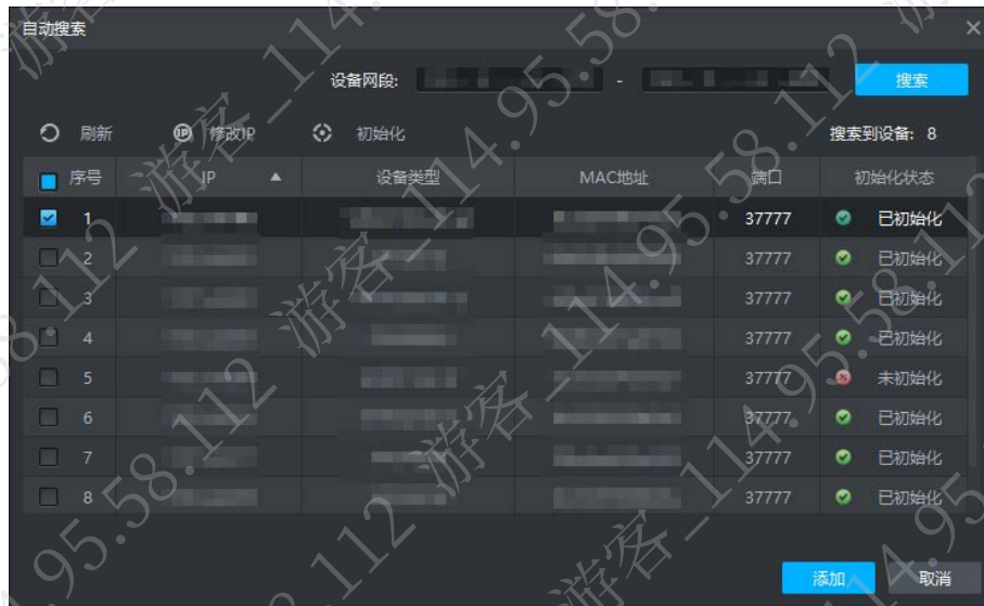
图1-5 自动搜索
