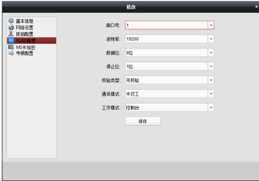
图6-22 RS485 配置框
