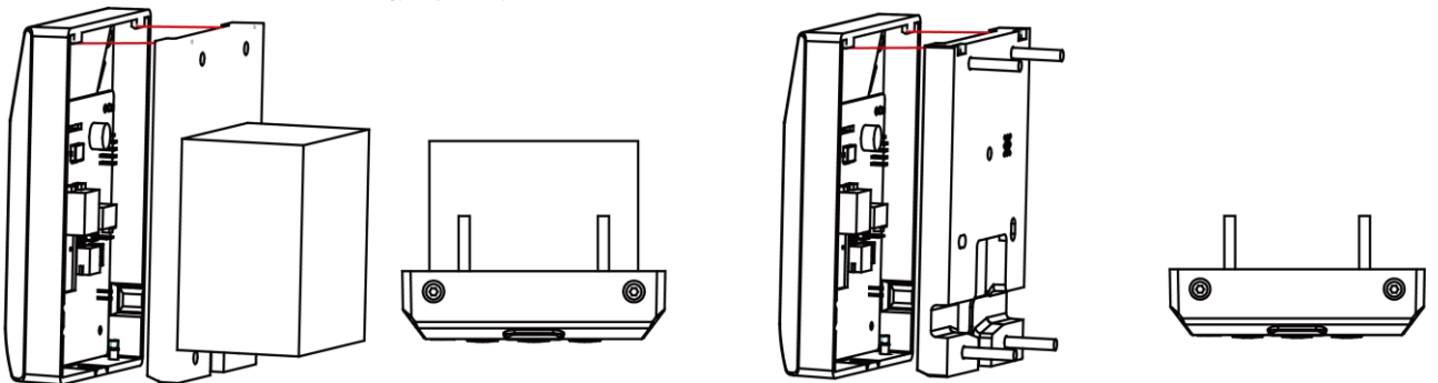
图3-3 锁住后壳
