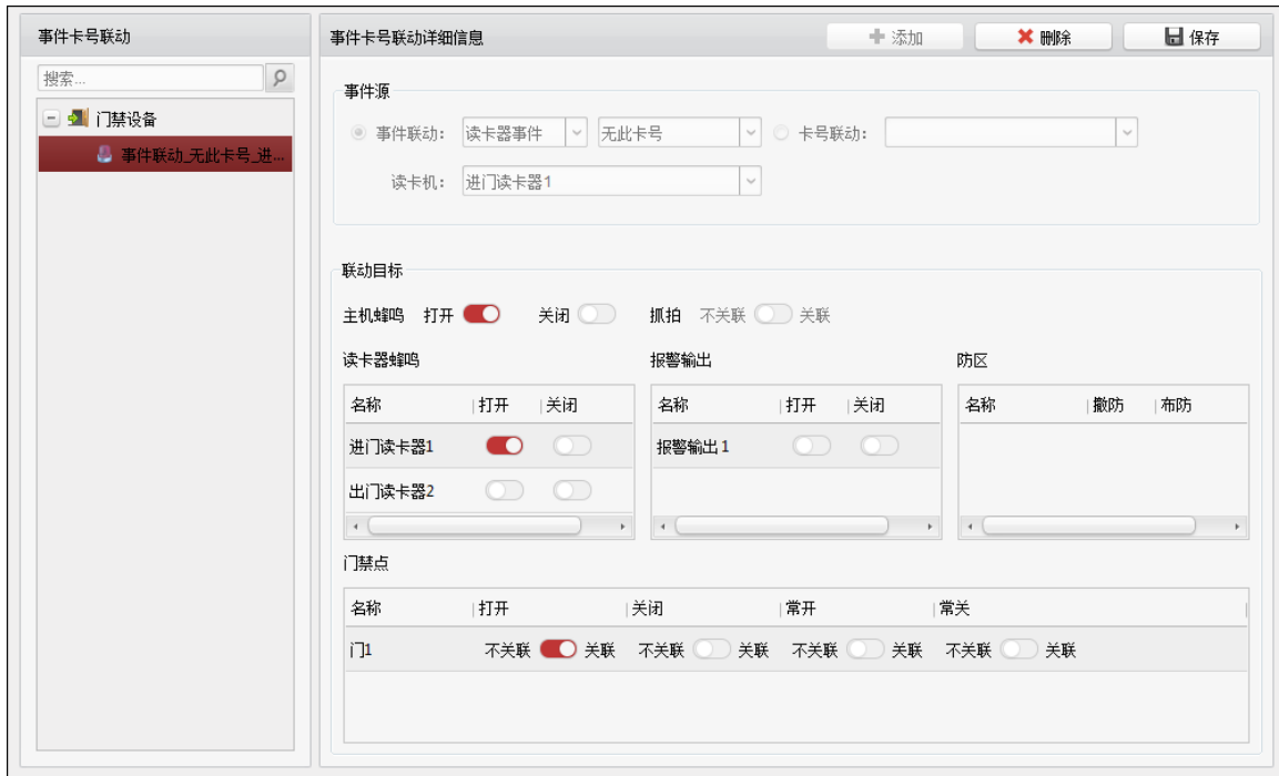
图6-111 事件卡号联动界面
