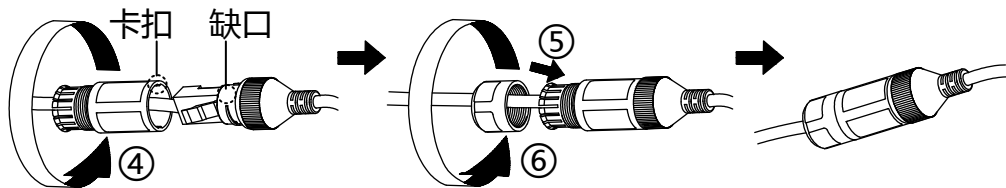
图1-9 完成安装
