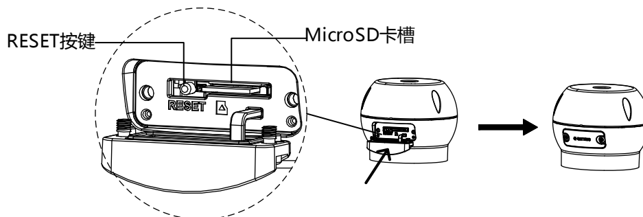
图1-2 安装 MicroSD 卡
