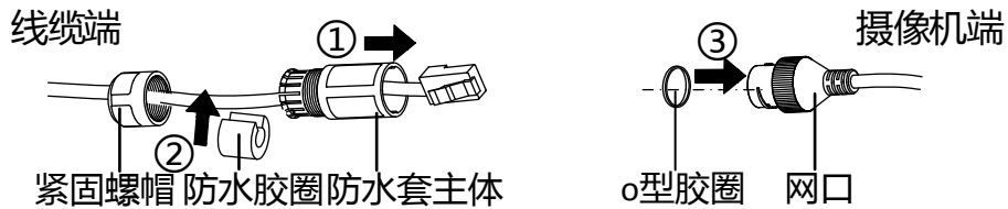
图1-8 安装网线
