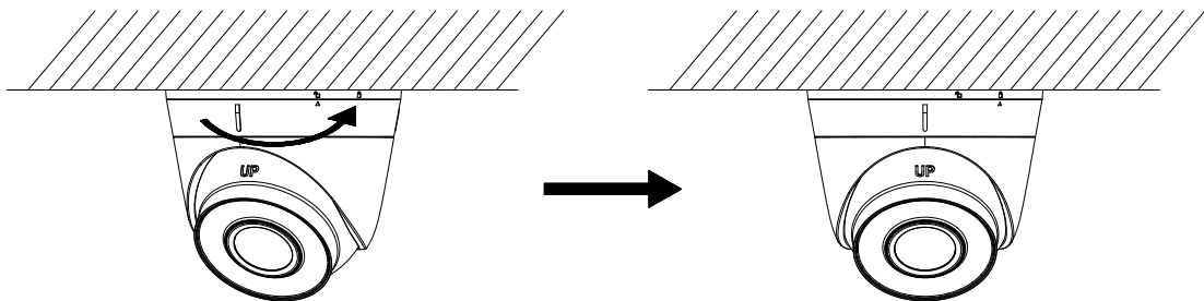
图1-4 安装摄像机
