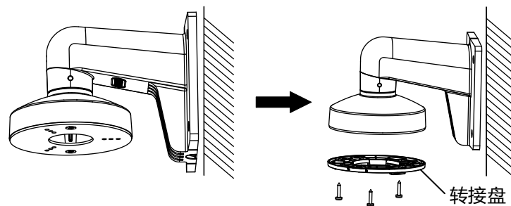
图1-6 安装壁装支架及转接盘
