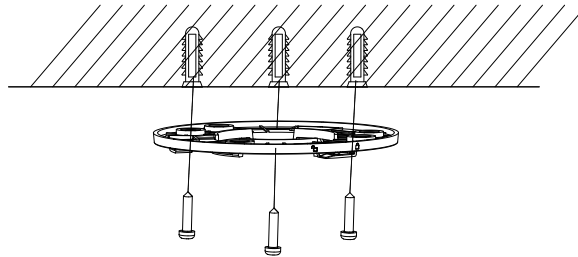
图1-3 安装转接盘
