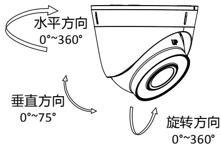
图1-5 调节角度
